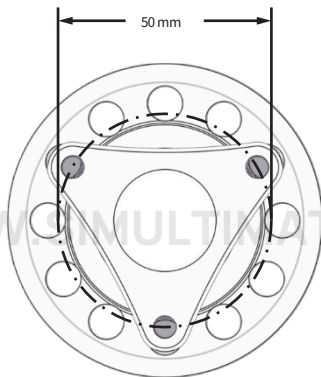
Diagramm der Befestigungslochpositionen
